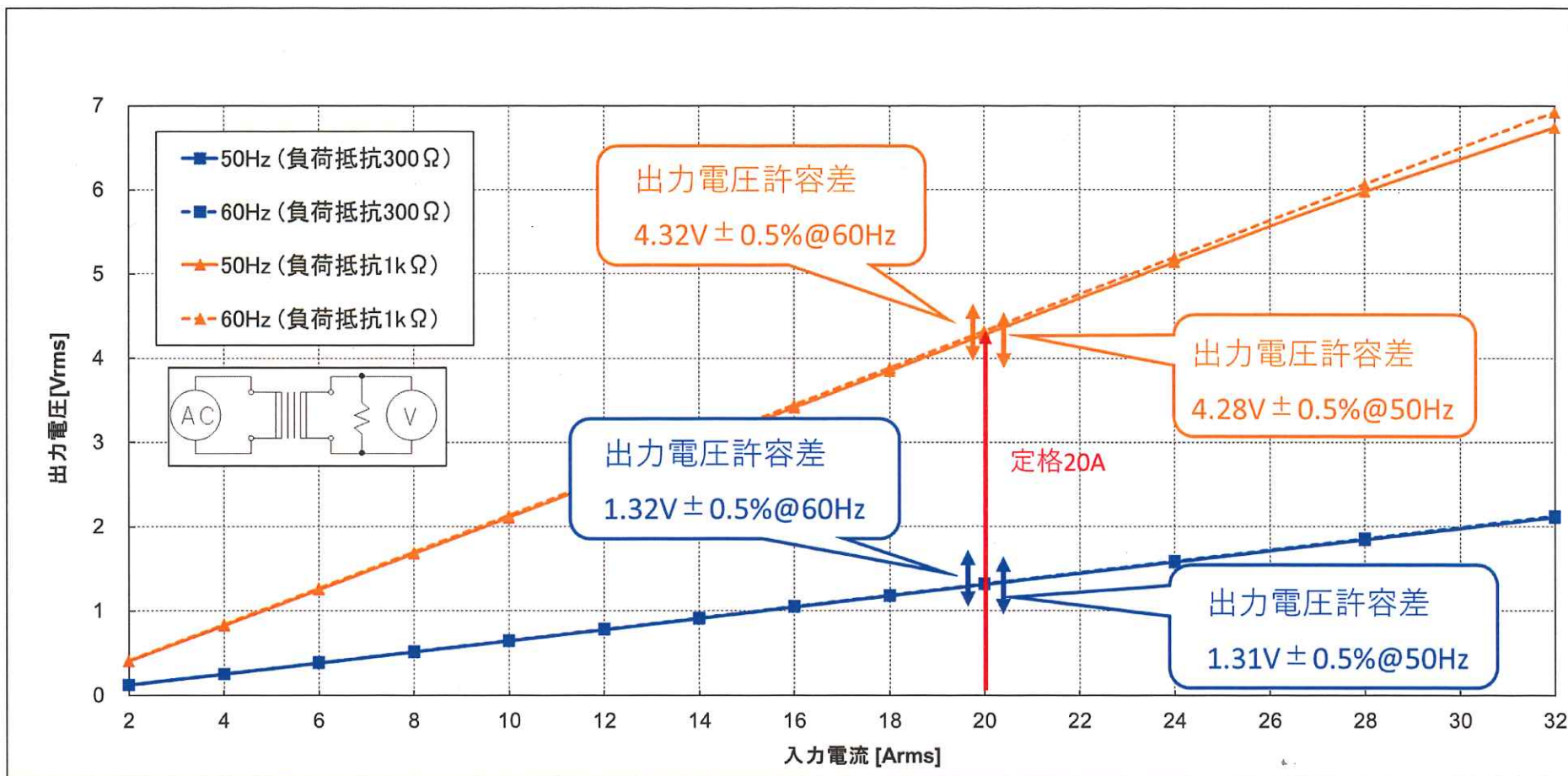
【グラフ1】 小型高精度カレントトランスEI-16H 電流-出力電圧特性例
