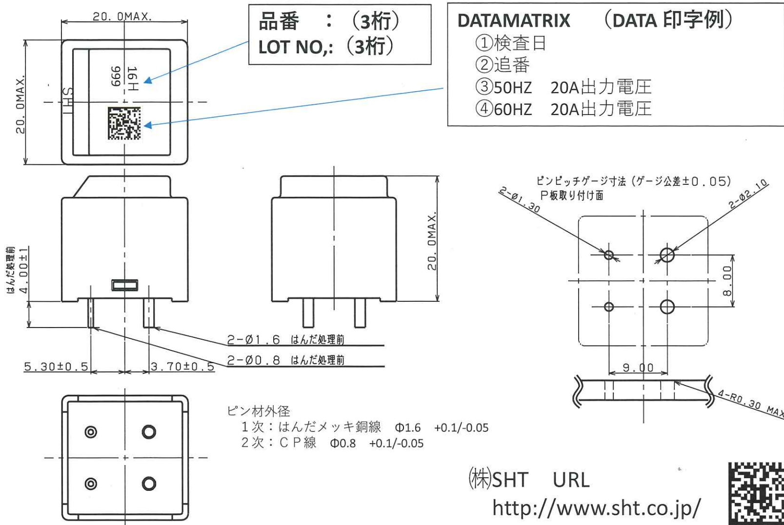
【図1】 小型高精度カレントトランスEI-16H 外観図 データマトリクス表示例
